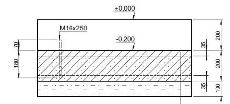
ZÁKL. DESKA / FOUNDATION BASEPLATE / FUNDAMENTPLATTE BETON / CONCRETE / BETONKLASSE C20/25, 200mm 2xKARISIT / MESH PANELS / BETONSTAHLMATTE - Ø 8, 150 x 150 ŠTĚRKOPÍSKOVÝ PODSYP / GRAVEL SUB-BASE / KIES UNTERGRUND, 100mm
