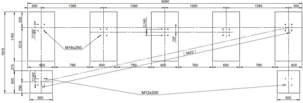
ZÁKLADOVÉ PATICE / BASE FOOTING / BETONFUSSFUNDAMENTE VAR B KUBATURA BETONU / CONCRETE CUBATURE / BETONRAUMINHALT - 2.28m 3
