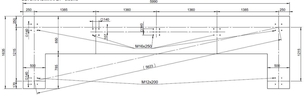
ZÁKLADOVÝ PAS / CONTINUOUS FOOTING / FUNDAMENTSTREIFEN VAR A KUBATURA BETONU / CONCRETE CUBATURE / BETONRAUMINHALT - 3.53m 3
